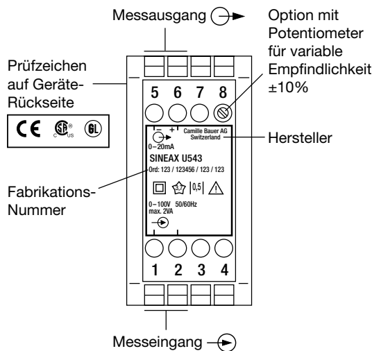
Bild 3. Erklärungen zum Typenschildbeispiel.
